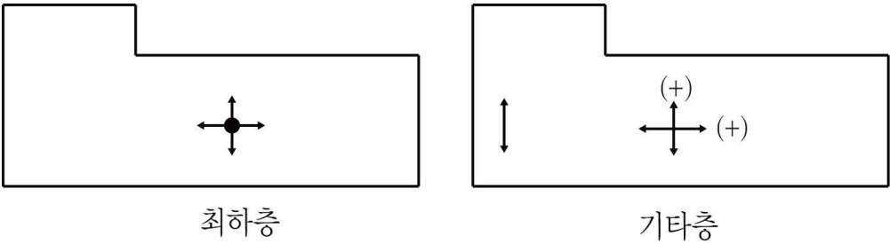
[별도 7] 비정형성이 적은 건축물의 지진가속도감지기 설치 위치 및 계측 성분(제15조 관련)
